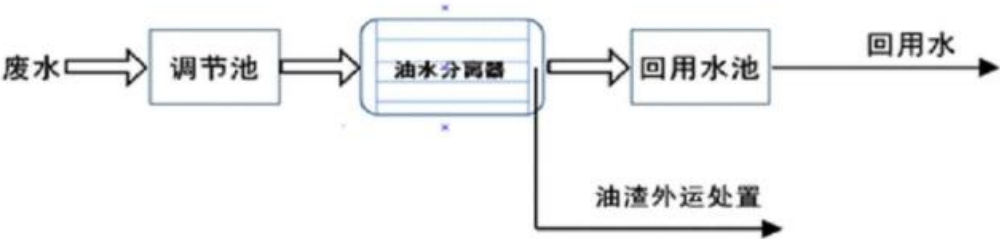
图 5-1 含油废水处理工艺流程图
